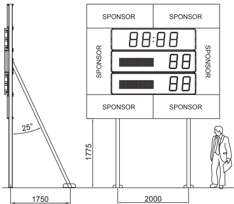
Support D (réf. 915174)
